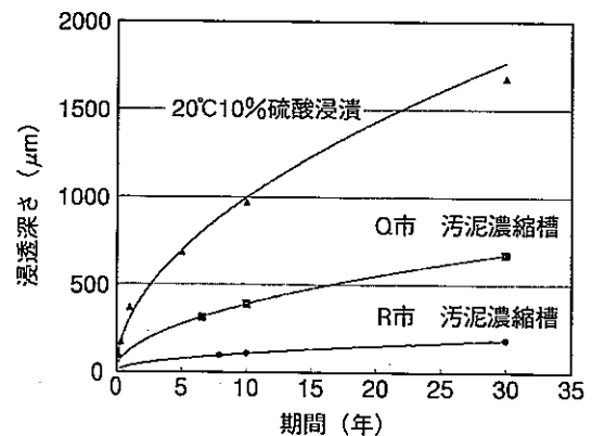
図-3 協会塗料化粧品 (H4) の硫黄侵入予測
