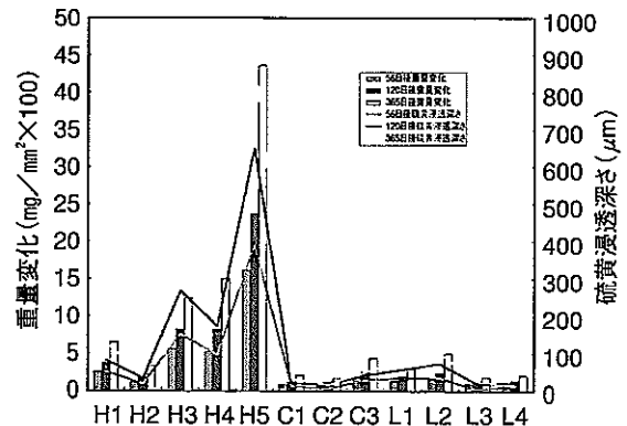
図-5 浸漬後の重量変化および硫黄侵入深さ
