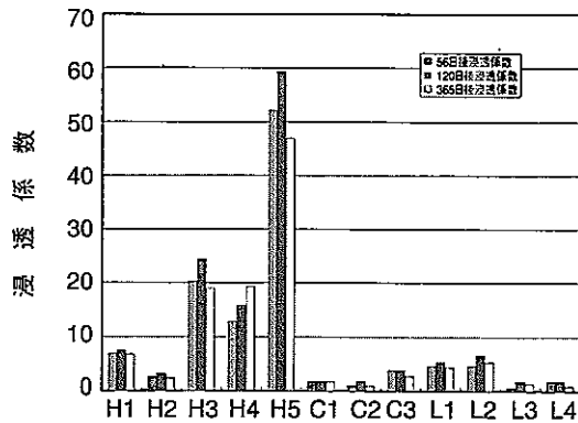
図-4 硫黄拡散係数 b ( \mu\text{m}/\sqrt{\text{日}} )
