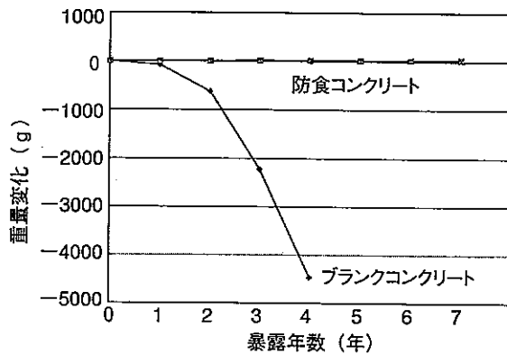
図-2 Q市汚泥濃縮槽における重量変化
