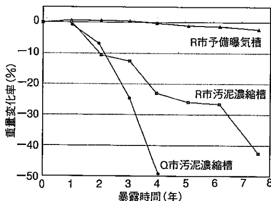
図-1 ブランクコンクリートの腐食状況
